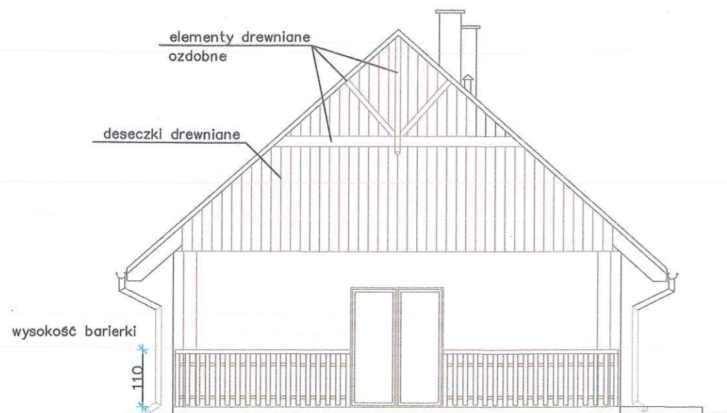
ELEWACJA POŁUDNIOWA
